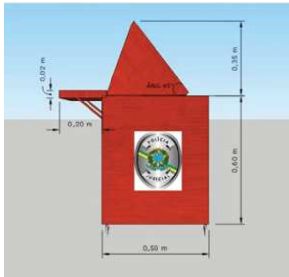
Imagem 4 – Vista lateral esquerda com cotas
