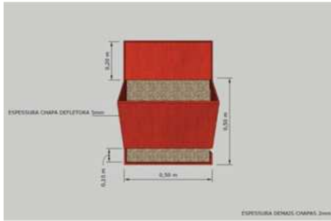
Imagem 3 – Vista topo com cotas
